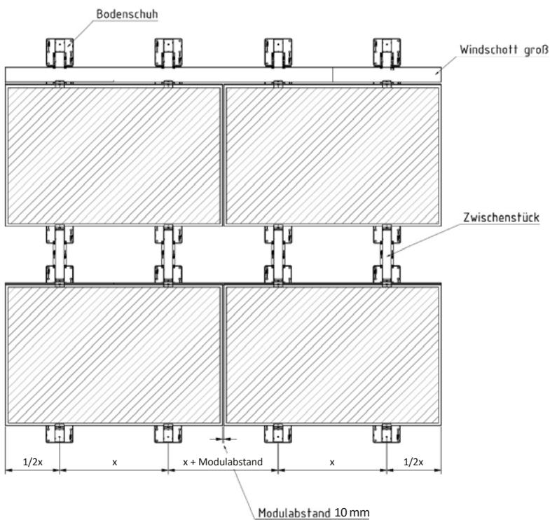
Abb.: 8.2b Aufmaß SL Fast Flat SÜD-System Viertelpunktklemmung
