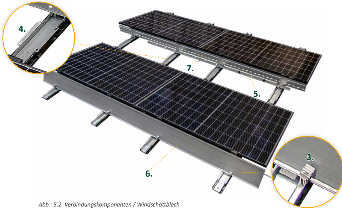
Abb.: 5.2. Verbindungskomponenten / Windschottblech
