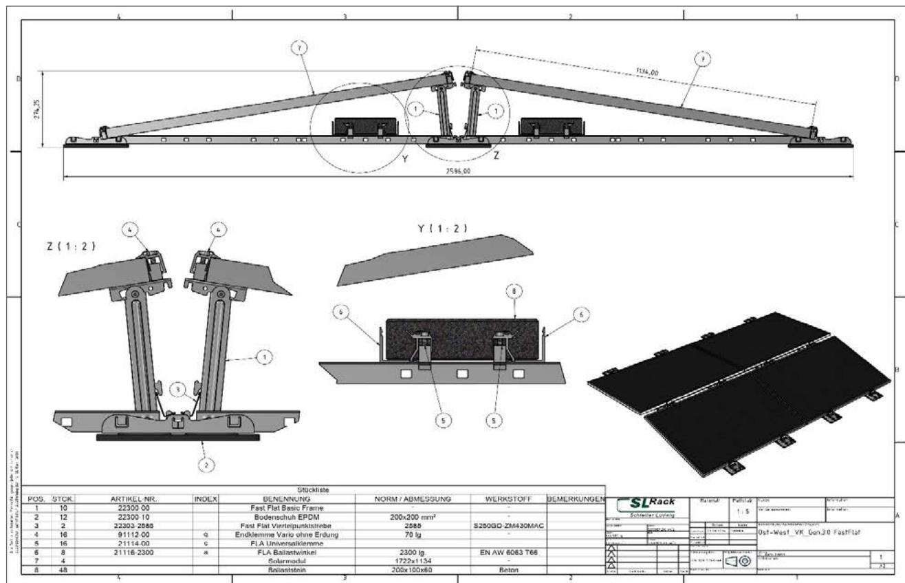
Abb.: 2.4. Beispiel SL Fast Flat
