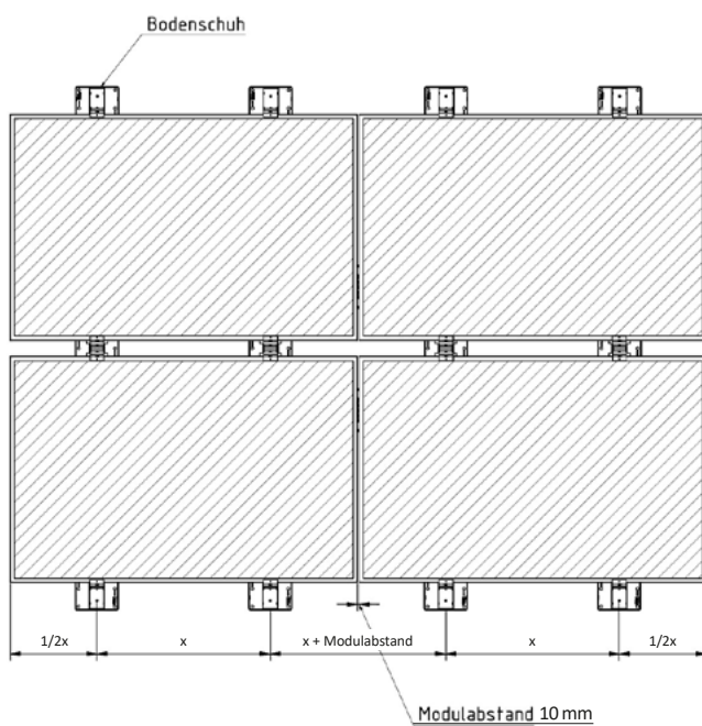
Abb. 8.2b Aufmaß OST/WEST
