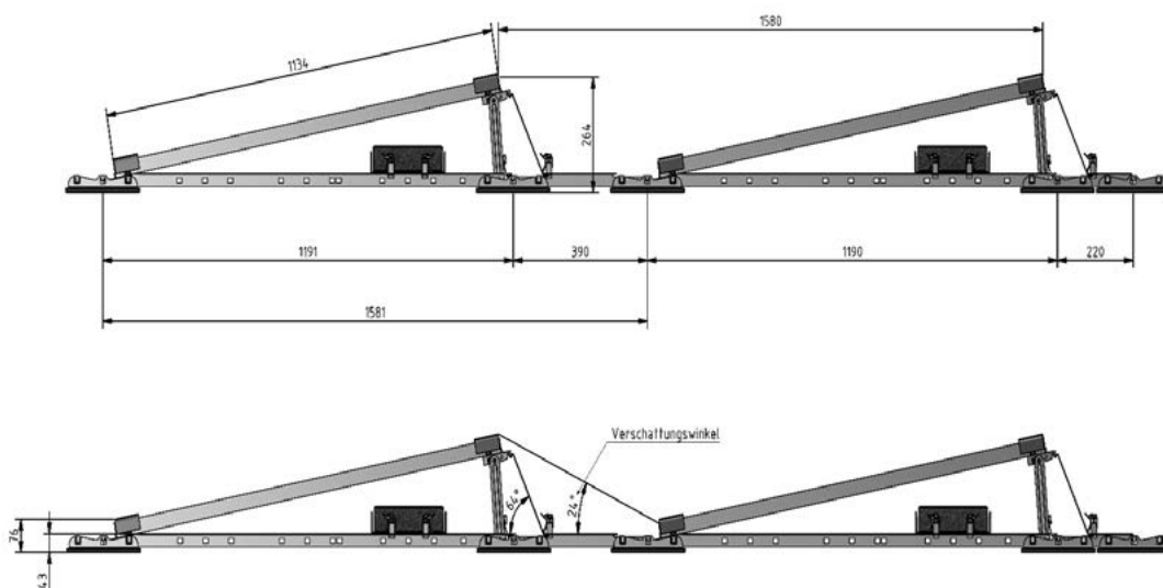
Abb.: 7.2. Beispielaufbau SÜD
